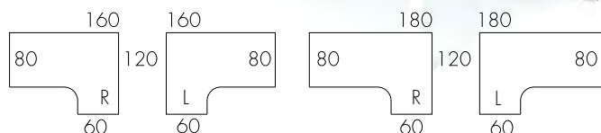
Compacte bladen 90°
